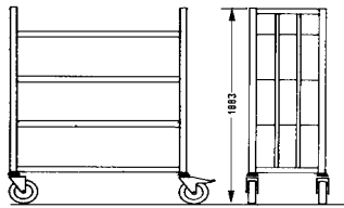
Regalwagen für Isoliertesgeschirr 600 x 1300 x 1883 80 Ober- oder 90 Unterteile
